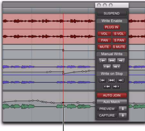
AutoJoin indicator
