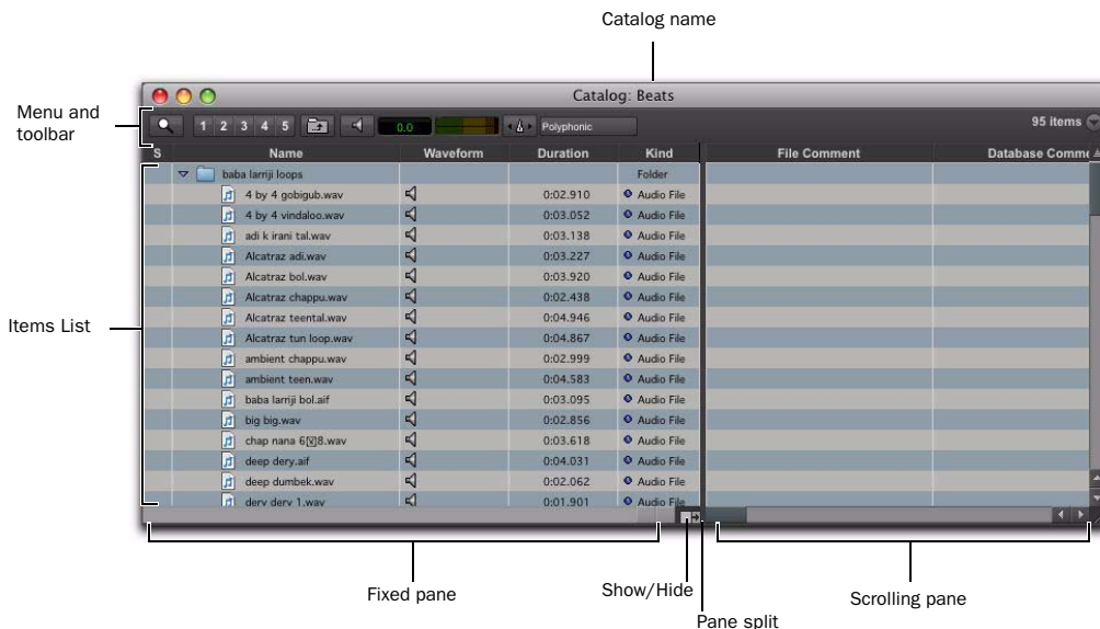
Figure 15. Catalog browser
