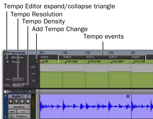
Tempo Editor
